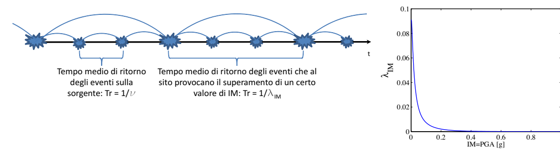
Figura 1. Concetto di filtraggio del PPO per passare dal processo di occorrenza dei terremoti nella sorgente al superamento dell'accelerazione al sito (sinistra); esempio di curva di pericolosità (destra).
