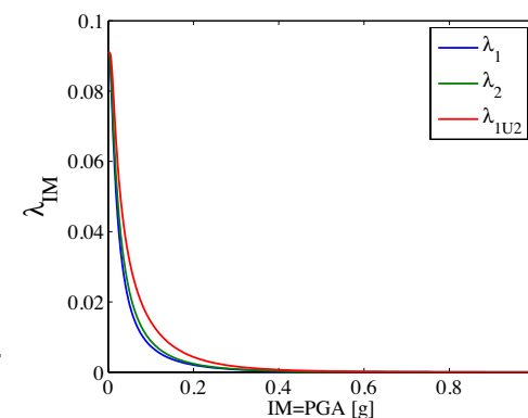
Figura 3 Siti 1 e 2 considerati nella zona sismogenetica 912 (sinistra) e curva della pericolosità dei due siti confrontata con la pericolosità sito-specifica (destra).
